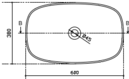
Vista dall'alto View from above Vista desde arriba Vue de dessus
