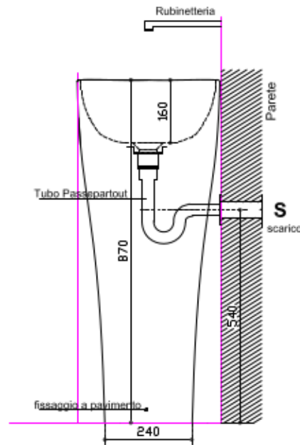
Vista laterale Lateral view Vista lateral Vue latérale
