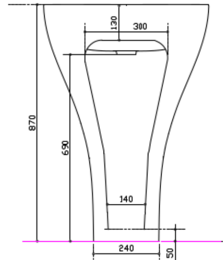
vista posteriore Back view Vista posterior Vue arrière
