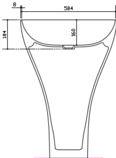
Sezione B-B Section B-B Sección B-B Section B-B
